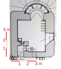
Žlebnik po Habrnál in drugi, sl. 200. Mali tipski objekt SdFTeJ - risbe tipov, lt. XI. ar. zb. = MT/14
