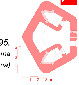
Žlebnik. Mali tipski objekt - " MT/P " (tip z eno prekucno oklepno strelno lino)
