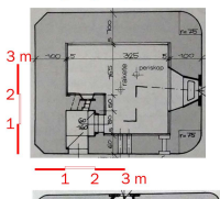
Habrnál in drugi, sl. 317. - UO za bočni ogenj Mali tipski objekt - " MT/MB "
