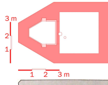
Žlebnik. Mali tipski objekt - " MT/P " (tip z eno prekucno oklepno strelno lino)
