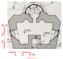
Habrnál in drugi, sl. 191. Mali tipski objekt - MT/7
