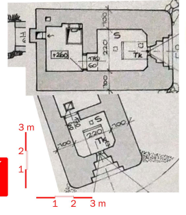
Habrnál in drugi, sl. 207. Mali tipski objekt - " MT/BL " (kota Blegoš)
